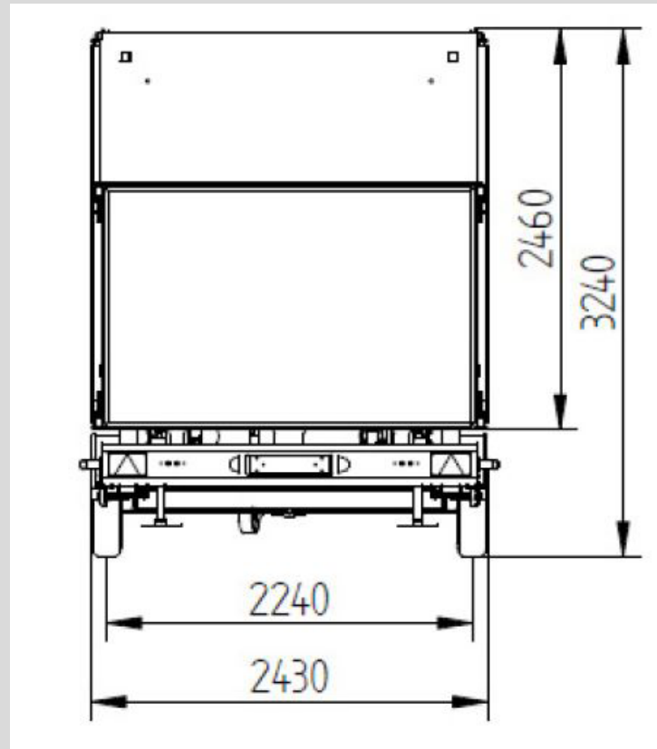
Transportmasse Anhänger
