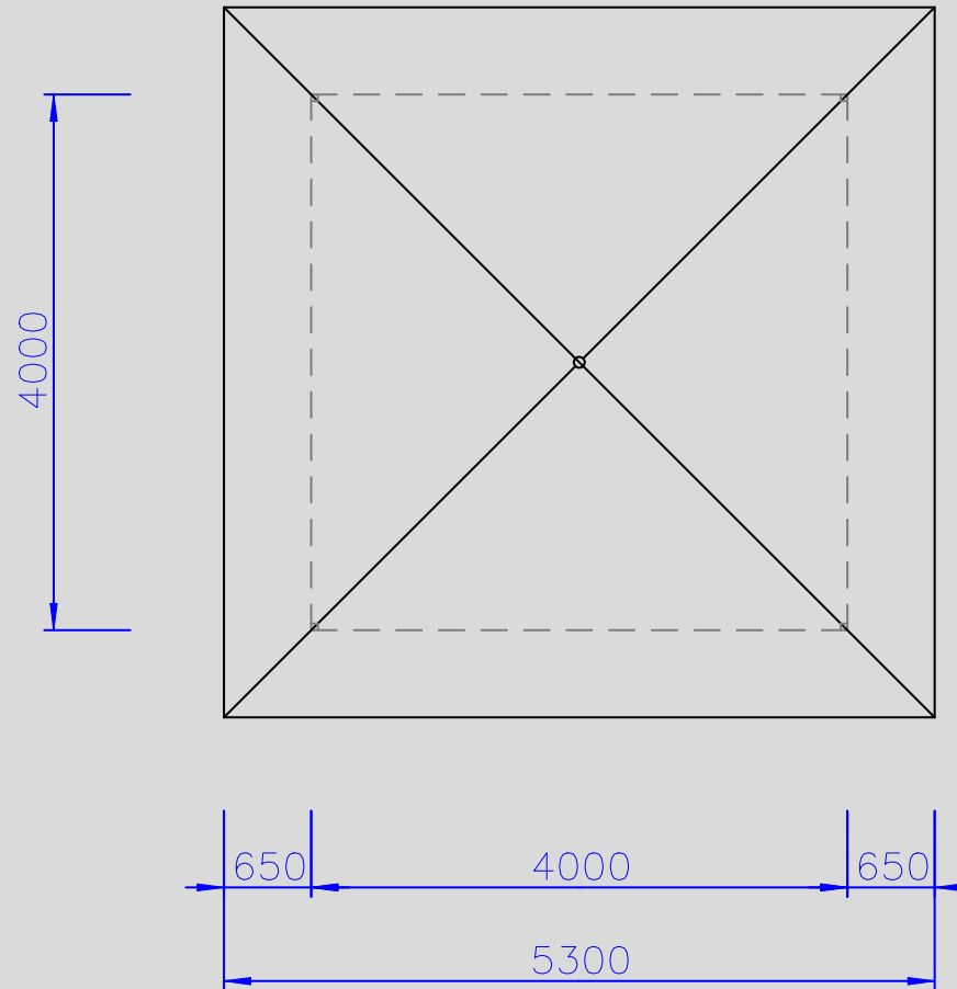
Draufsicht
